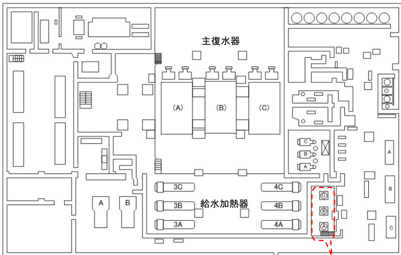
給水加熱器ドレンポンプ3台の位置
